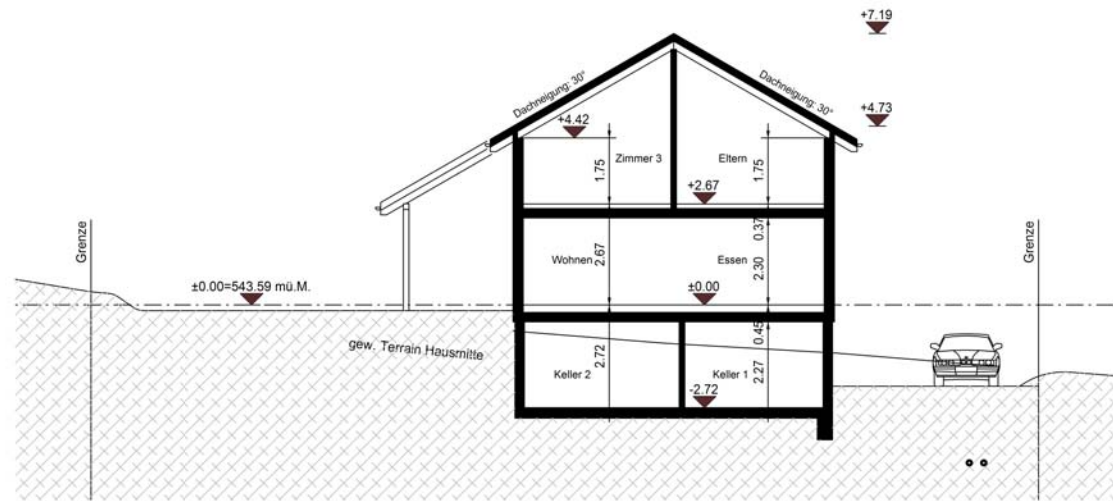
Querschnitt
