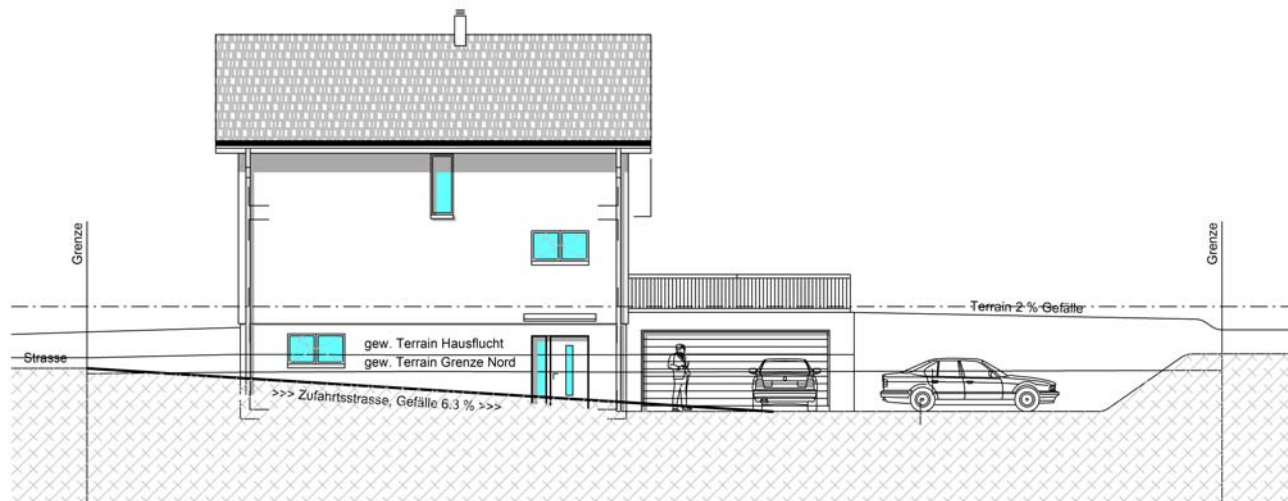
Ansicht Nordfassade
