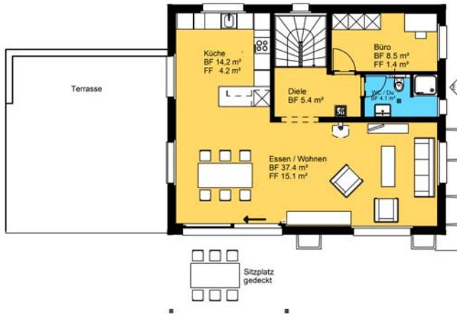
Erdgeschoss
