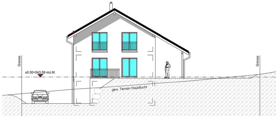
Ansicht Westfassade
