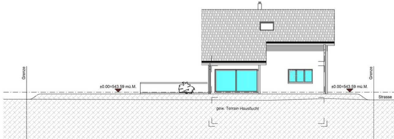
Ansicht Südfassade
