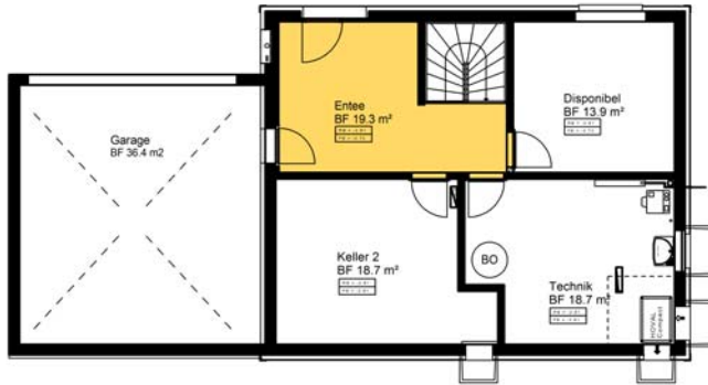
Untergeschoss
